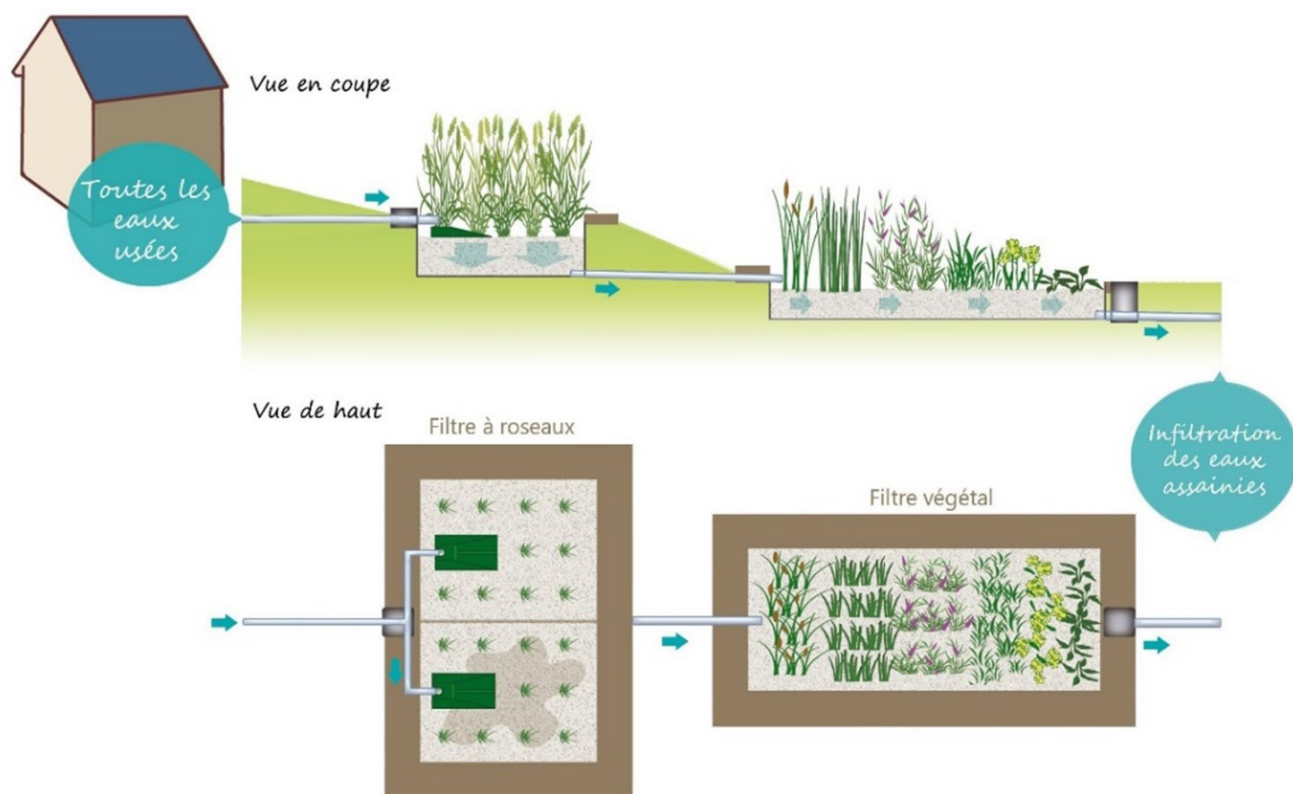
Schéma simplifié du Jardin d'Assainissement® IRIS
