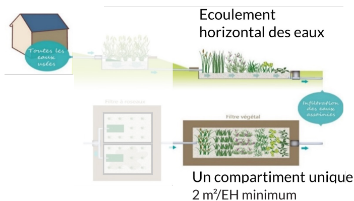
Schéma simplifié du filtre à écoulement horizontal = filtre végétal
