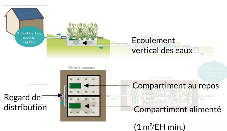
Schéma simplifié du filtre à écoulement vertical = filtre à roseaux
