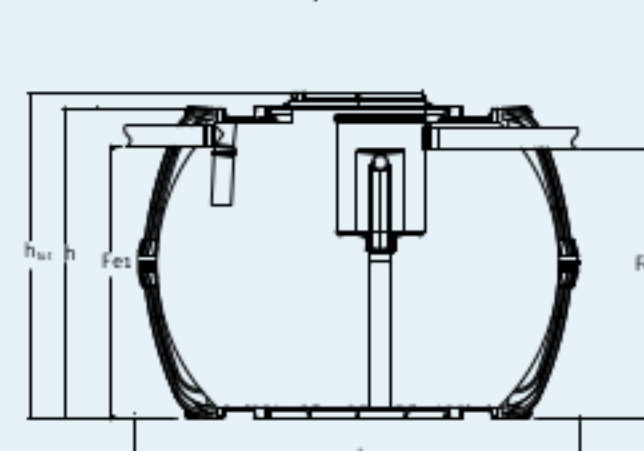
Fosses toutes eaux Carat super renforcées
