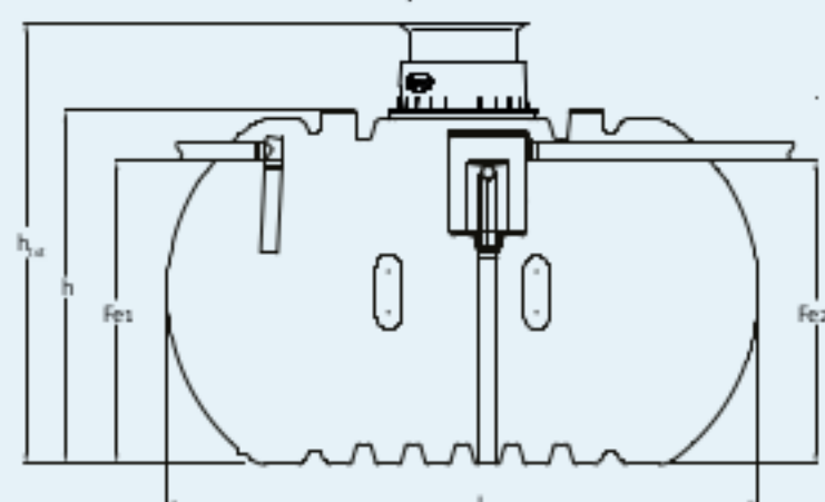
Fosses toutes eaux Carat XL super renforcées
