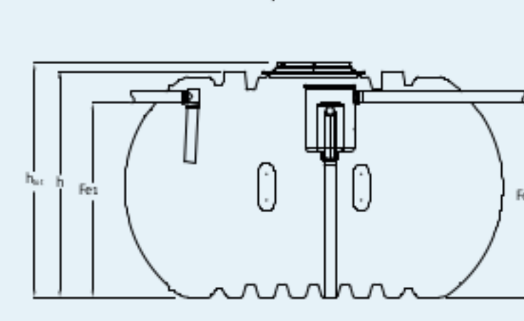
Fosses toutes eaux Carat XL super renforcées
